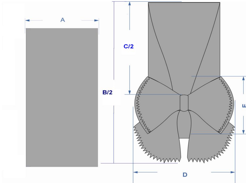
FIGURA 1 DIMENSIONES BANDA
