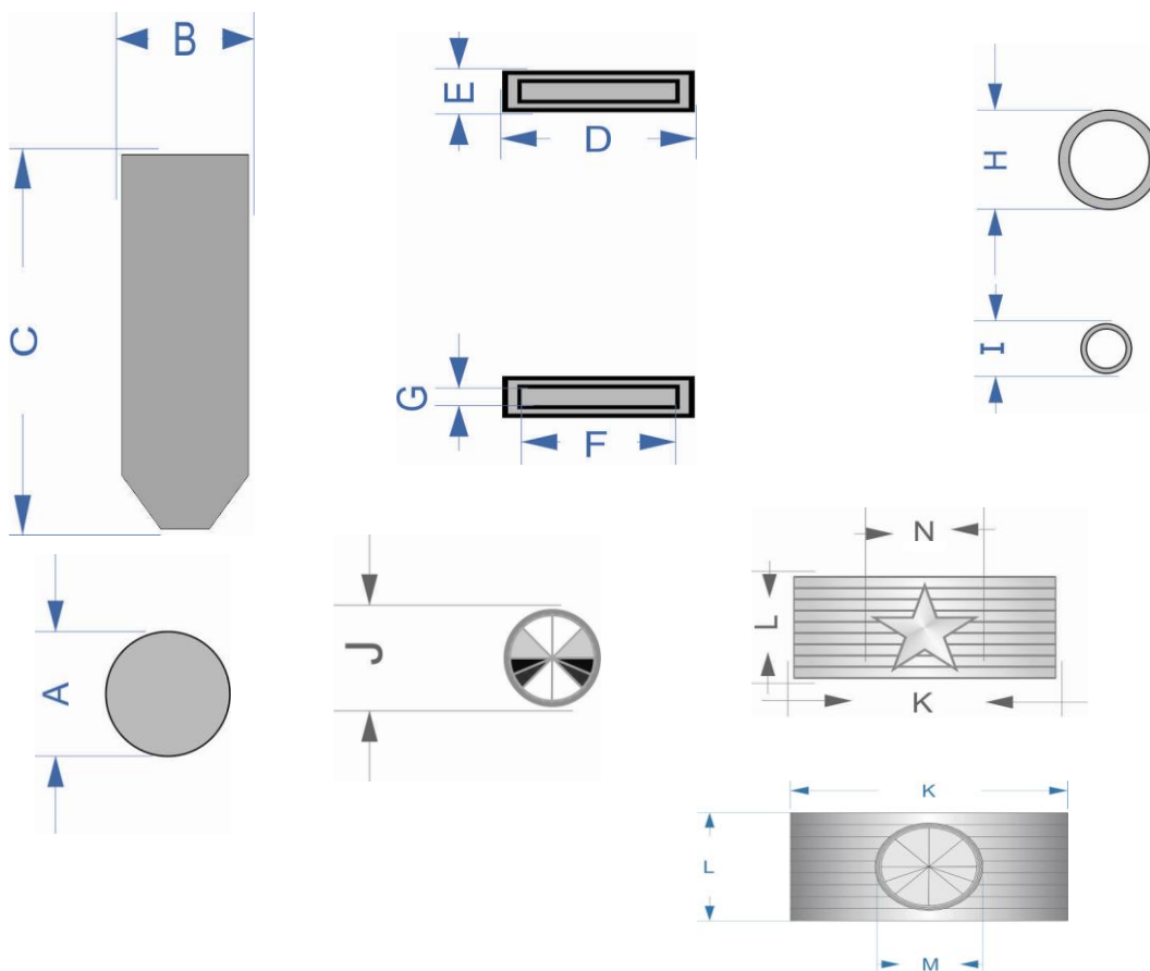
FIGURA 3 DIMENSIONES REPLICA
