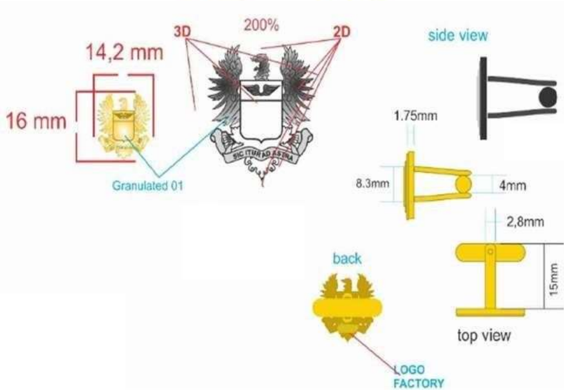
Figura 11. Dimensiones MANCORNAS
