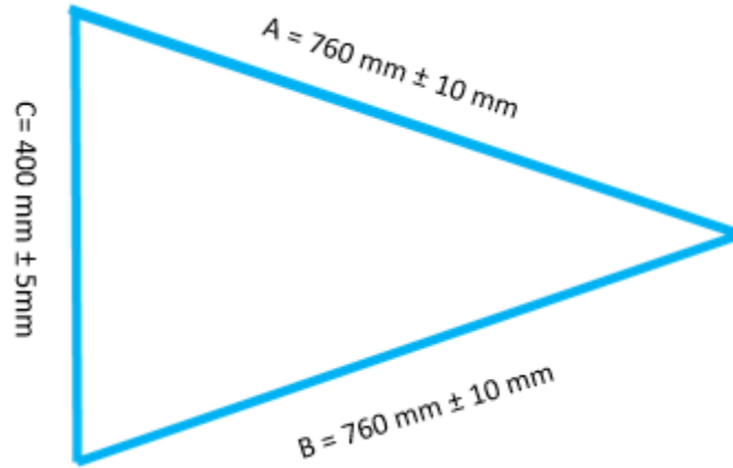
FIGURA 12. DIMENSIONES BANDERIN
